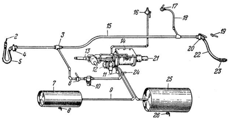
Рис. 2. Схема будови гальма типу PM [1, фіг. 657, С. 720]
